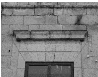
Izquierda: Figura 25. Enlace de dovelas de platabanda y jambas de marco de ventana con muro de sillares, casa del cura Juan Bruno de Luna. Derecha: Figura 26. Capialzado de piedra de cantería aparejada concéntricamente, que enlaza a los dos paramentos del muro. Palacio Episcopal.
