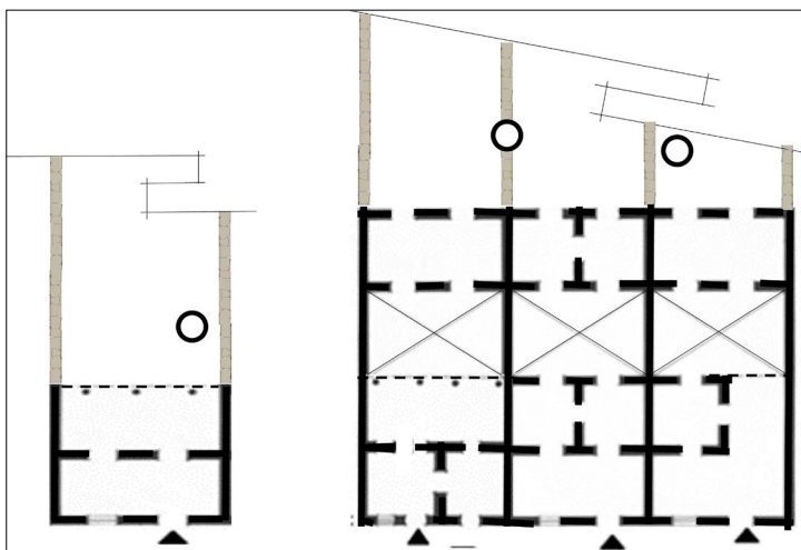
Figura 9. Plantas arquitectónicas de vivienda popular colonial para clase social baja, siglos XVI y XVII. 195
