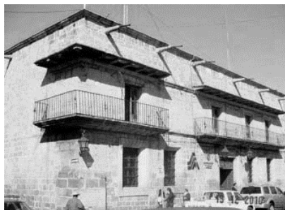
Izquierda: Figura 28. Vanos de puertas y ventanas a plomo unos sobre otros, casa del cura Juan Bruno de Luna.
