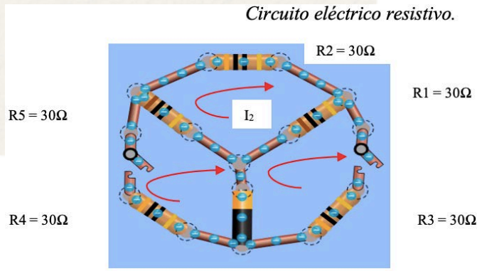
Figura 4. Circuito eléctrico resistivo.
