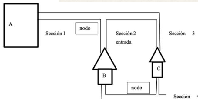
Figura 3. Alimentación de dos depósitos a través de un tanque de agua.
