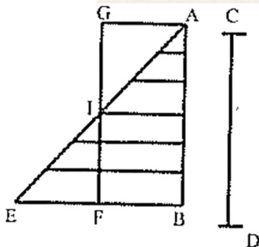
Figura 3. Construcción geométrica del teorema
