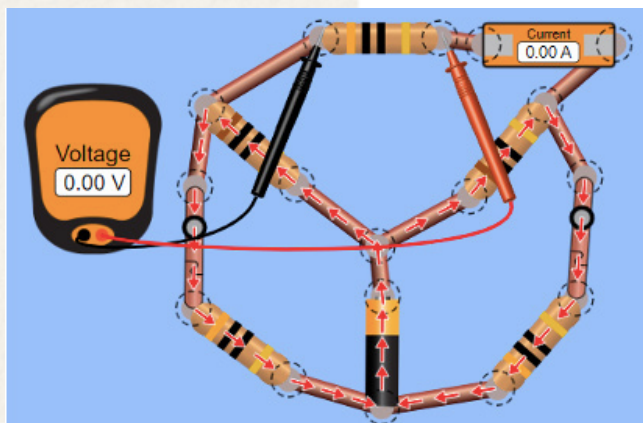
Figura 8. Circuito eléctrico resistivo elaborado por los participantes
