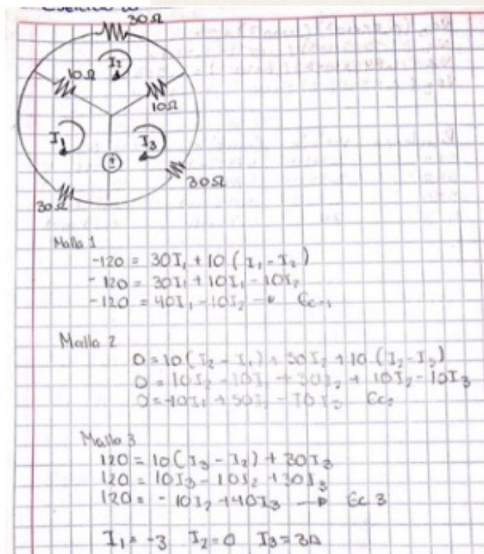
Figura 9. Obtención de las ecuaciones del análisis del circuito resistivo
