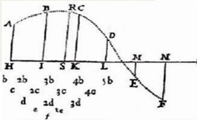
Figura 4. Escrito original de Newton: diferencias sucesivas
