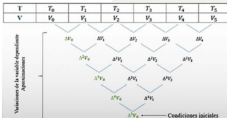
Figura 19. Diferencias de las diferencias
